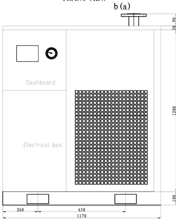
WIDOK Z PRZODU FRONT VIEW
