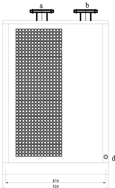
WIDOK Z LEWEJ LEFT VIEW
